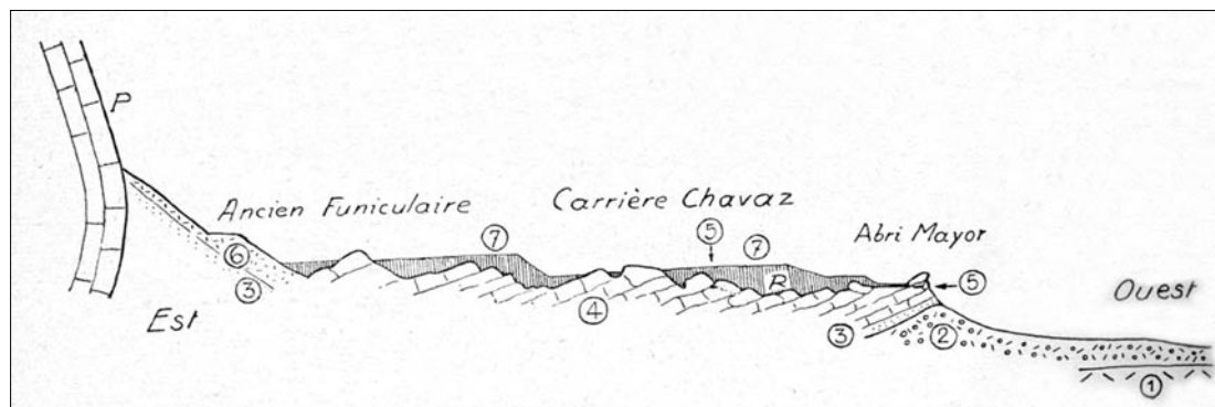
Fig. 14 Coupe générale synthétique publiés par Adrien Jayet en 1943. 1 : glacière würmien. 2 : moraine latérale. 3 : groise. 4 : masses calcaires écroulées. 5 : foyers magdaléniens et Magdalénien en place. 6 : éboulis. 7 : remblais.
